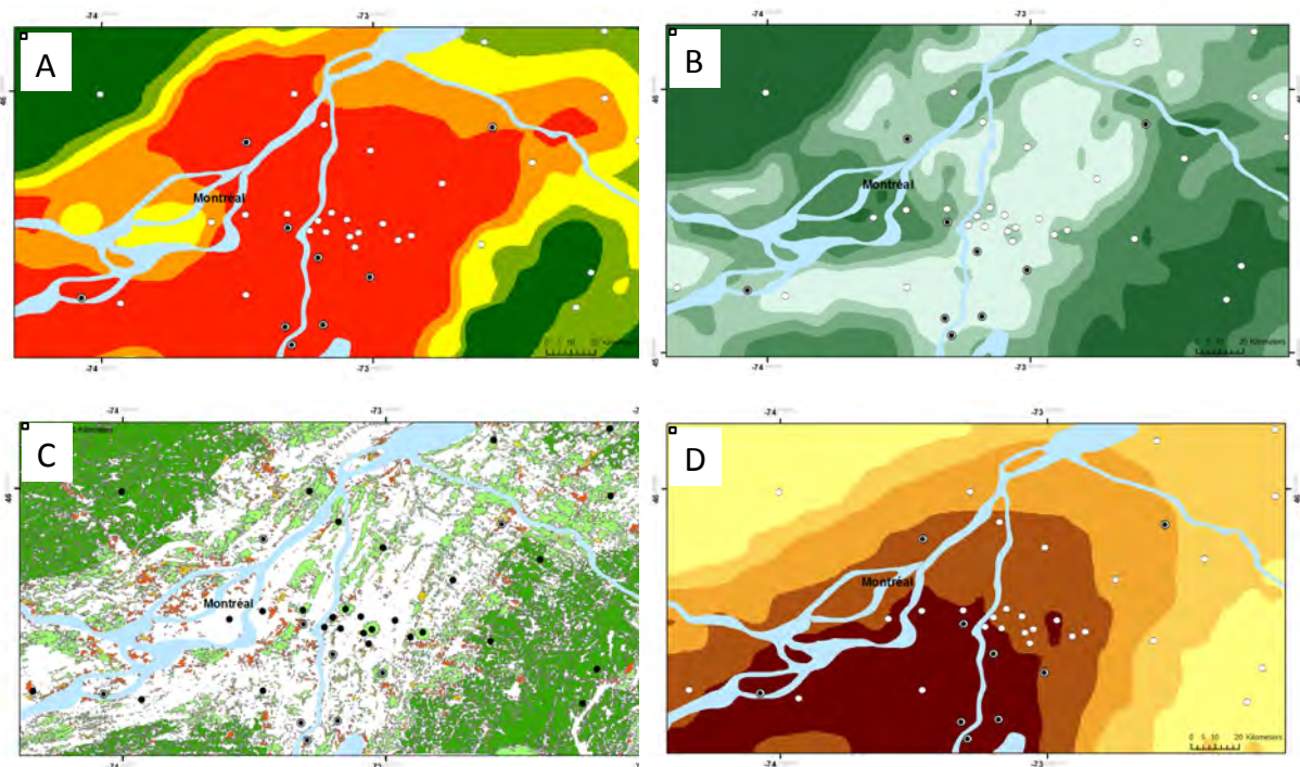
Figure 10. Les différentes couches utilisées pour modéliser la probabilité de présence de B. burgdorferi dans notre zone d'étude ; A : modèle climatique de niche de la souris à pattes blanches (la probabilité de présence varie de 0 en vert foncé à 1 en rouge) ; B : index de qualité de l'habitat pour la souris à pattes blanches (les zones en vert pâle sont des zones agricoles et les zones en vert foncé sont des forêts) ; C : degré de connectivité de l'habitat variant du rouge (isolé) au vert foncé (connecté) ; D : probabilité de présence de la tique I. scapularis selon le modèle de Ogden et al. (2008).
