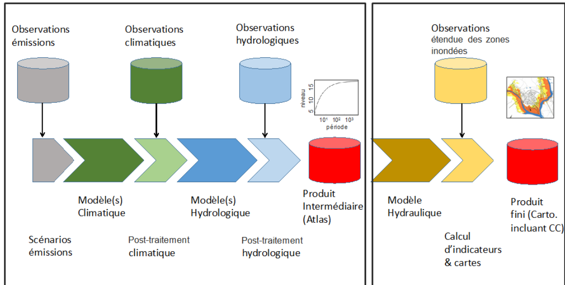
Figure 1. Chaîne de modélisation hydroclimatique (adapté de Dottori et al. 2016). À gauche, les éléments faisant partie de la portée des travaux de la thématique.
